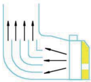
Рис. 4.2. Направление воздуха от радиатора отклоняющими лопастями
